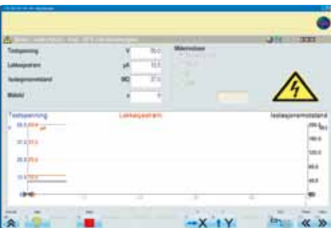
Isolasjonsmåling
