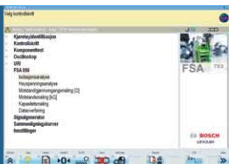
FSA oppstartsmeny
